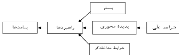
نمودار ۱: الگوی پارادایم در کدگذاری محوری (محقق ساخته)
